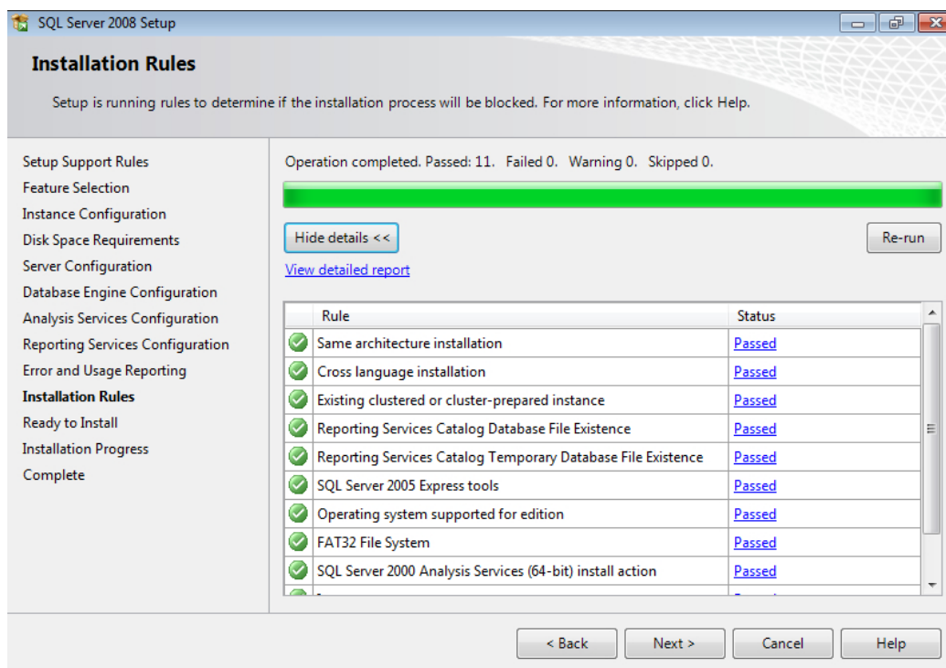
Рисунок 196. Раздел Installation Rules
