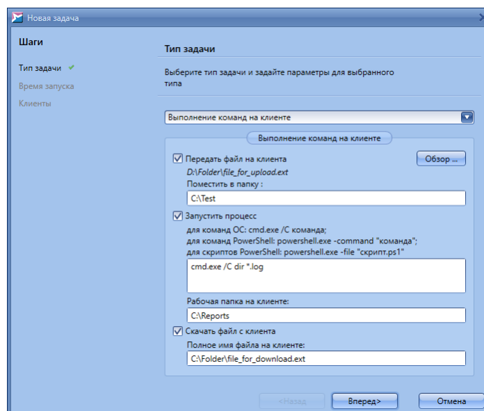
Рисунок 123. Шаг «Тип задачи»
