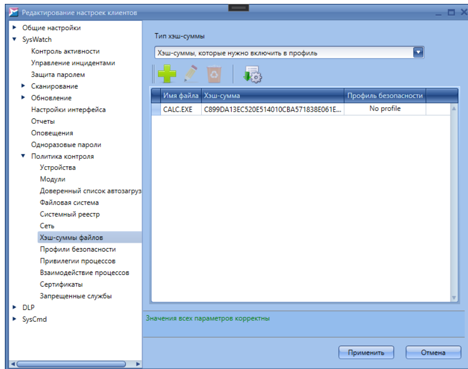
Рисунок 86. Хэш-суммы файлов
