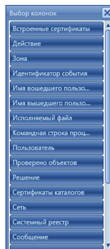
Рисунок 138. Выбор колонок
