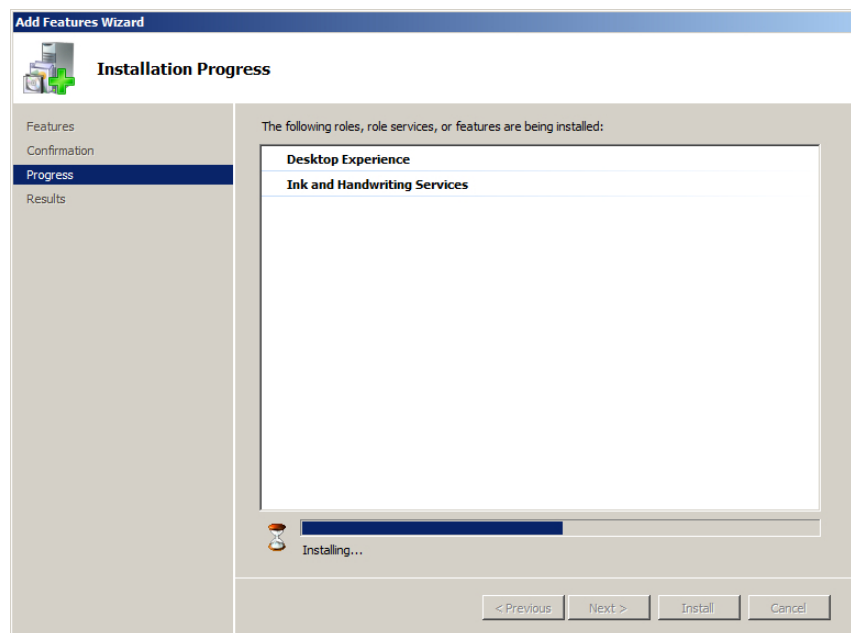
Рисунок 205. Процесс установки
