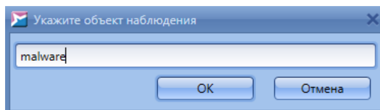
Рисунок 105. Объект наблюдения
