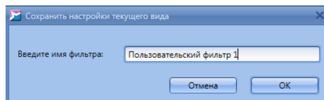
Рисунок 143. Сохранение фильтра
