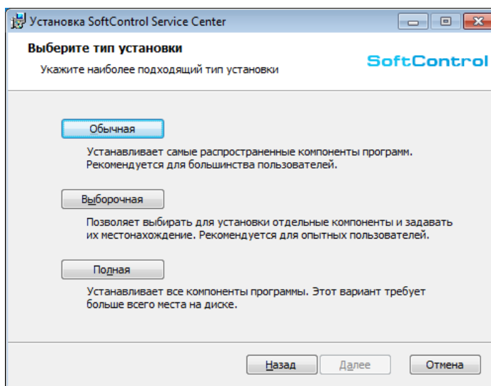
Рисунок 9. Типы установки
