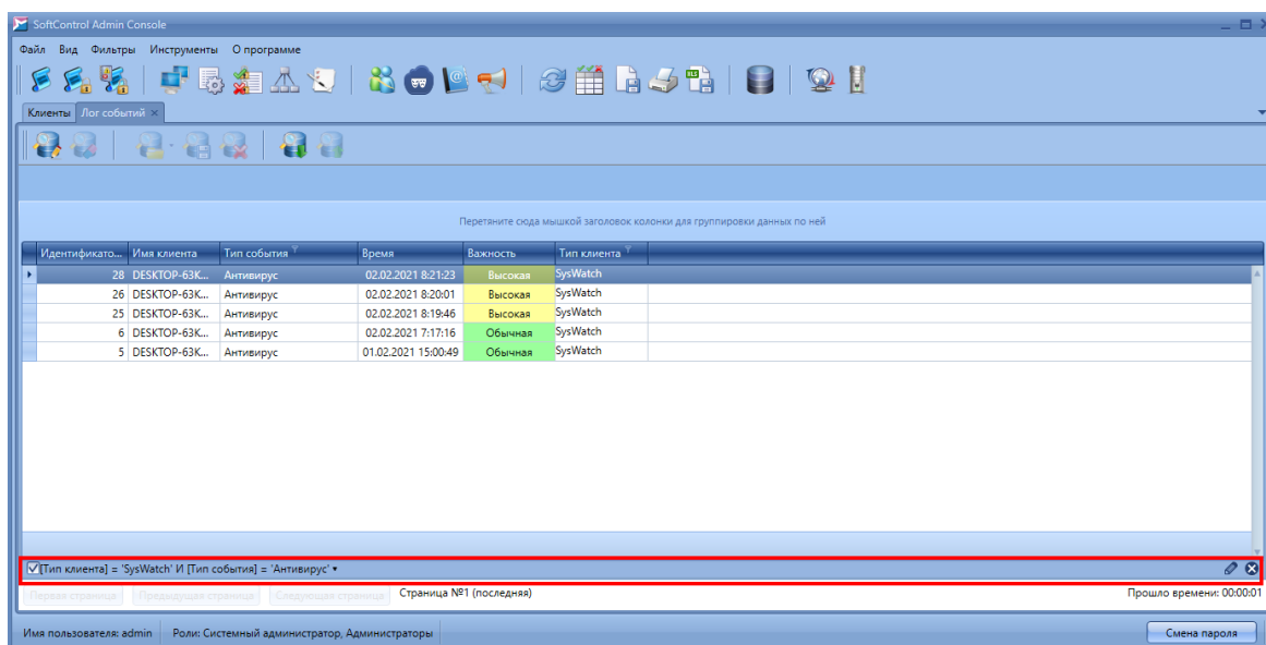
Рисунок 140. Настроенный фильтр
