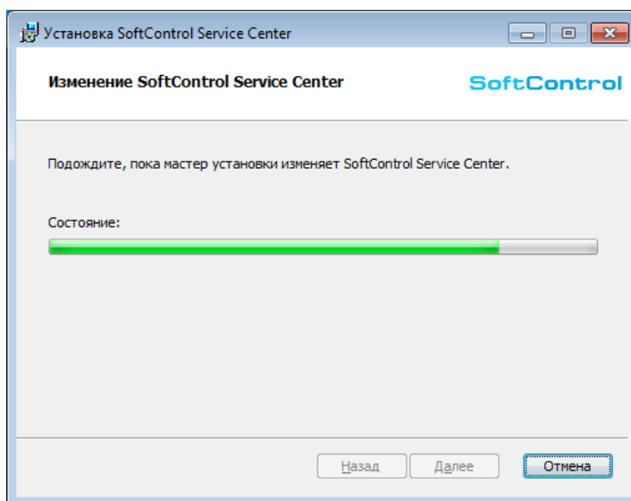
Рисунок 176. Процесс удаления
