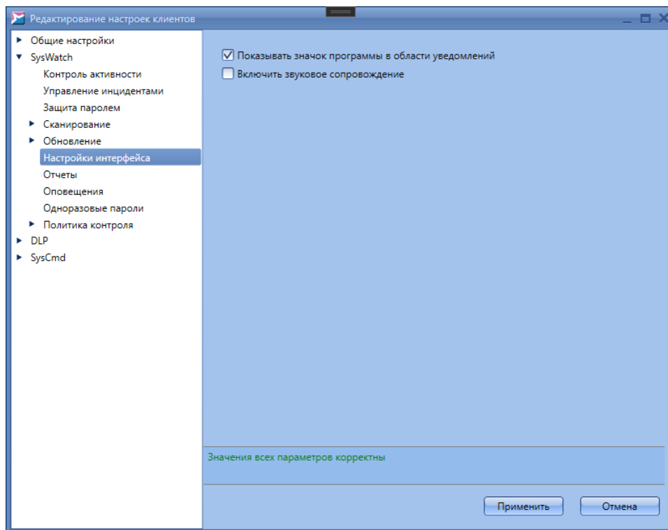
Рисунок 66. Настройки интерфейса
