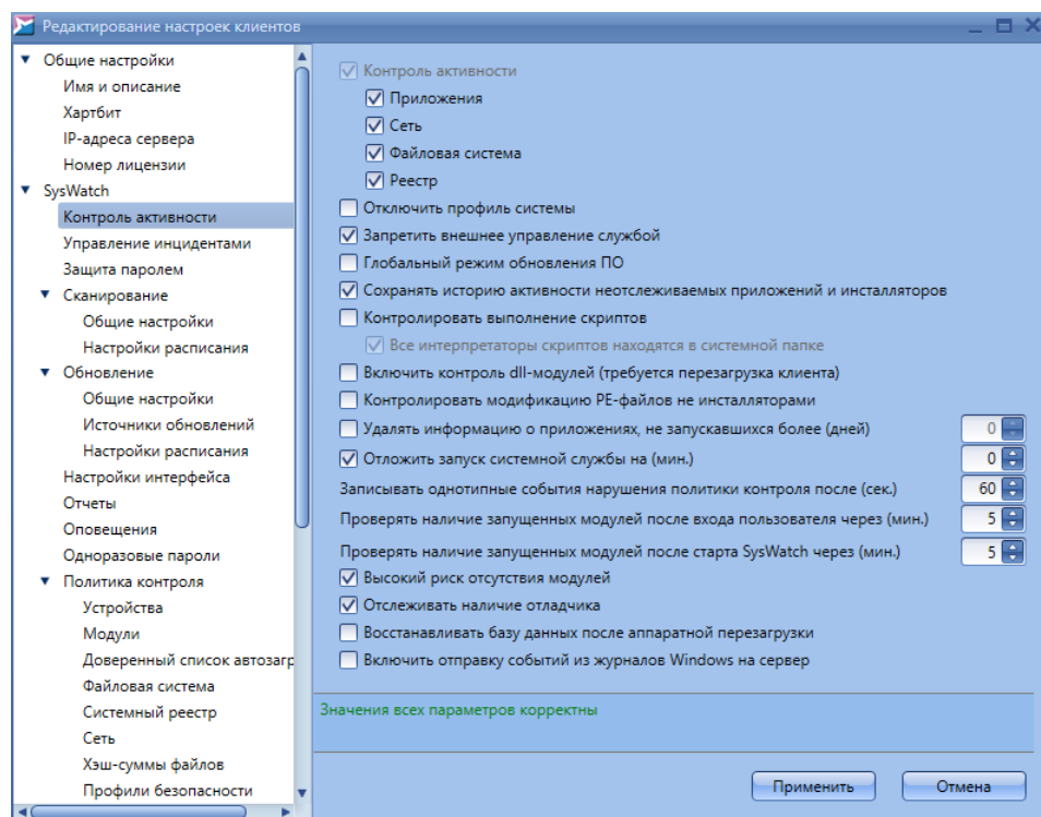
Рисунок 58. Настройки контроля активности
