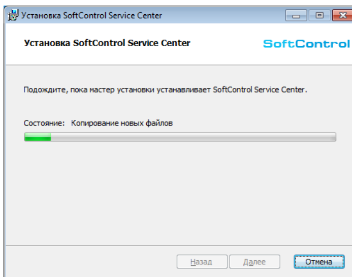
Рисунок 5. Процесс установки
