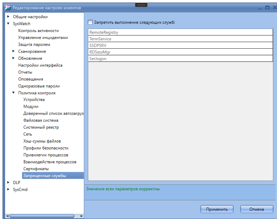
Рисунок 97. Запрещенные службы
