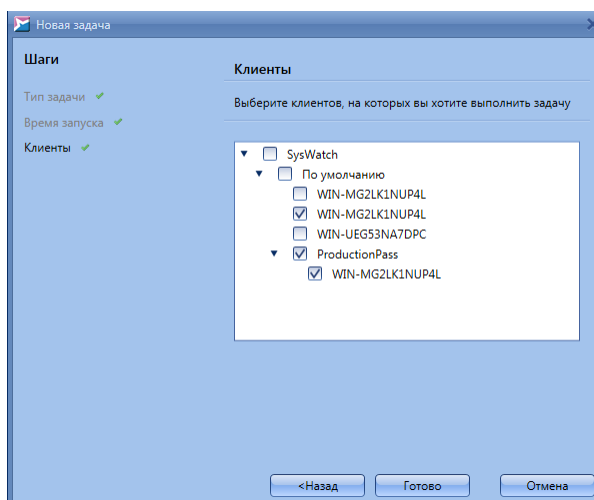
Рисунок 115. Шаг «Клиенты»
