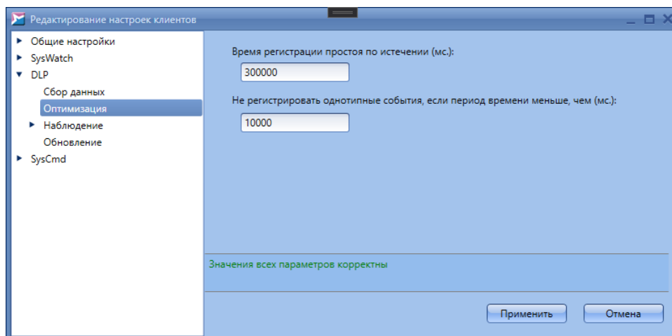
Рисунок 99. Настройки оптимизации
