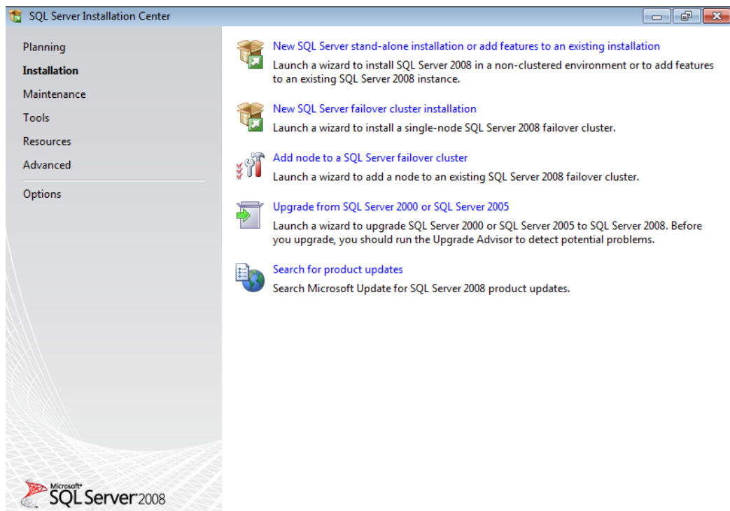
Рисунок 178. Раздел Installation
