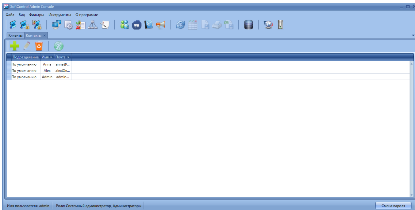
Рисунок 149. Вкладка «Контакты»
