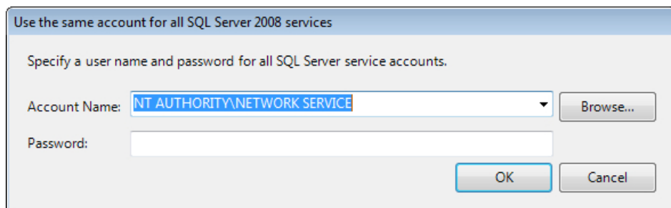
Рисунок 188. Учетная запись
