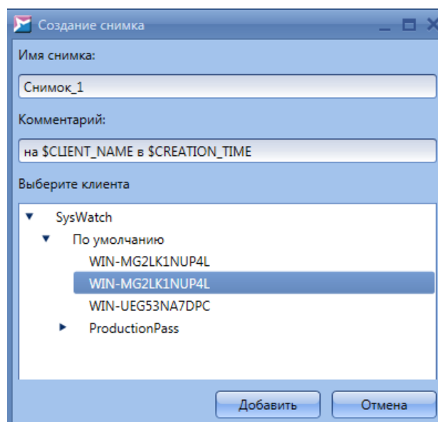
Рисунок 160. Создание снимка
