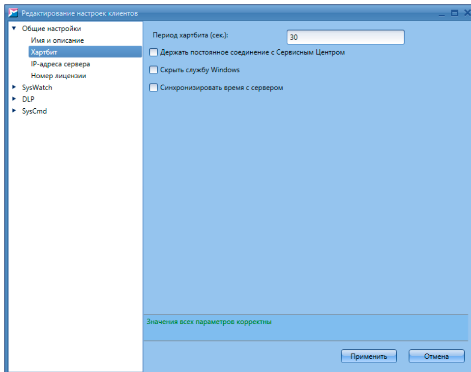
Рисунок 55. Раздел «Хартбит»
