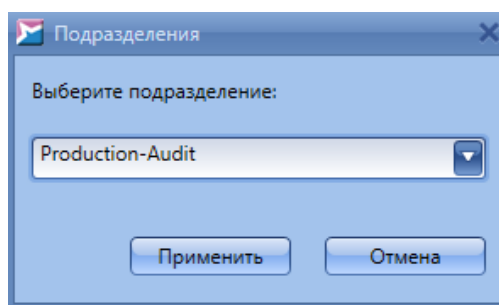
Рисунок 47. Перемещение подразделения
