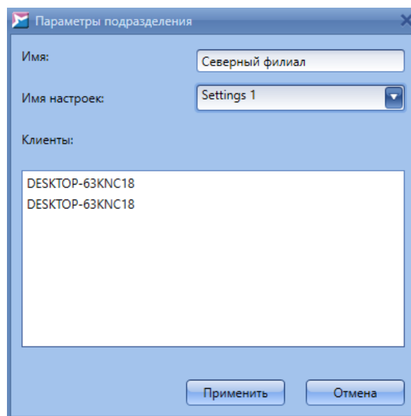
Рисунок 46. Параметры подразделения
