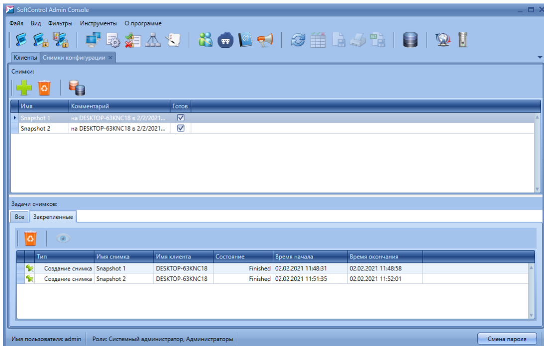
Рисунок 162. Закрепленные задачи
