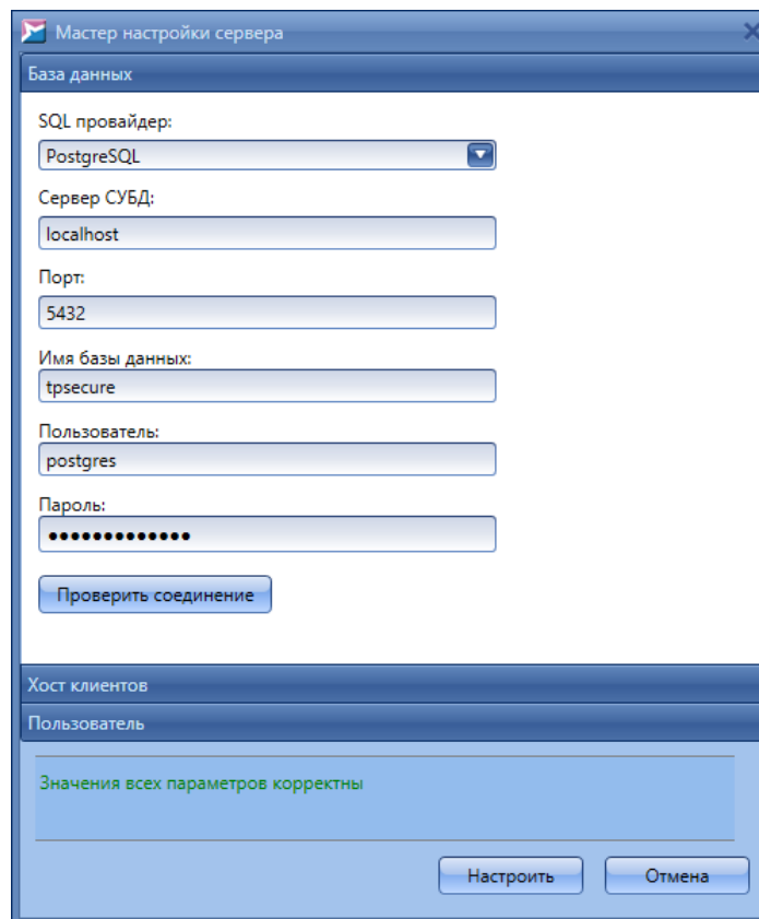
Рисунок 23. Настройка подключения к СУБД PostgreSQL
