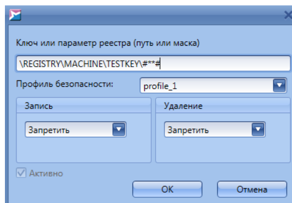
Рисунок 81. Создание правила для объекта системного реестра
